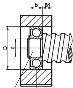
ukončení šroubu S5-d
