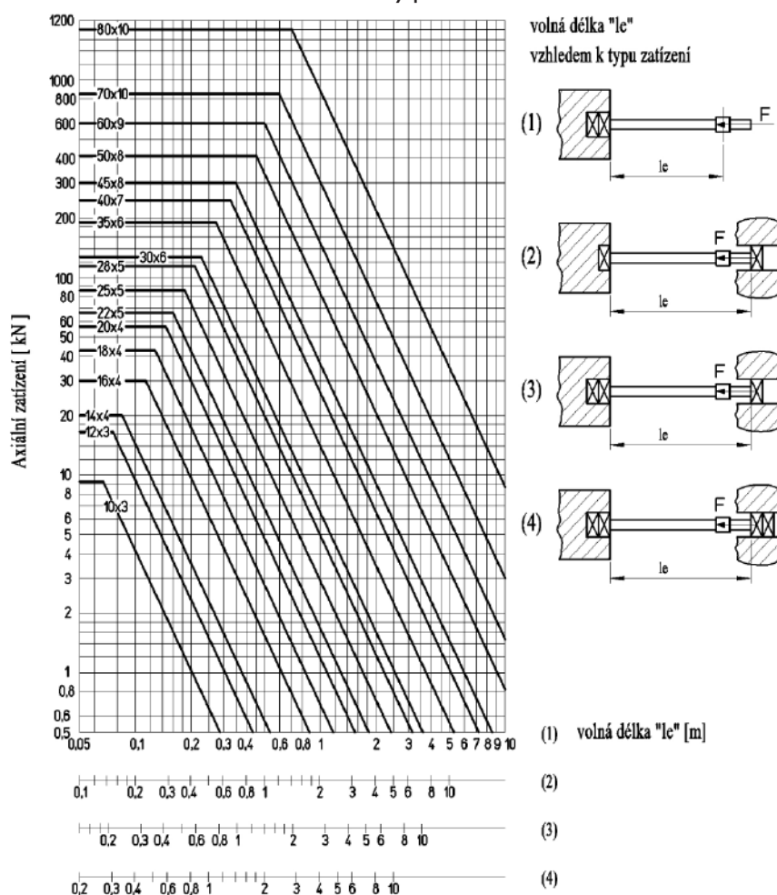
Graf č. 7: Kritický počet otáček
