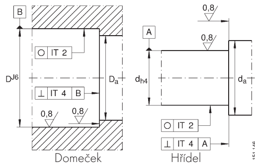
Tolerance pro ložisko ZKLN...2RS/ZZ
